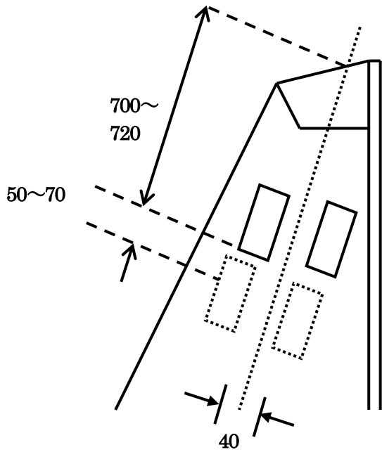
<国際470級>
