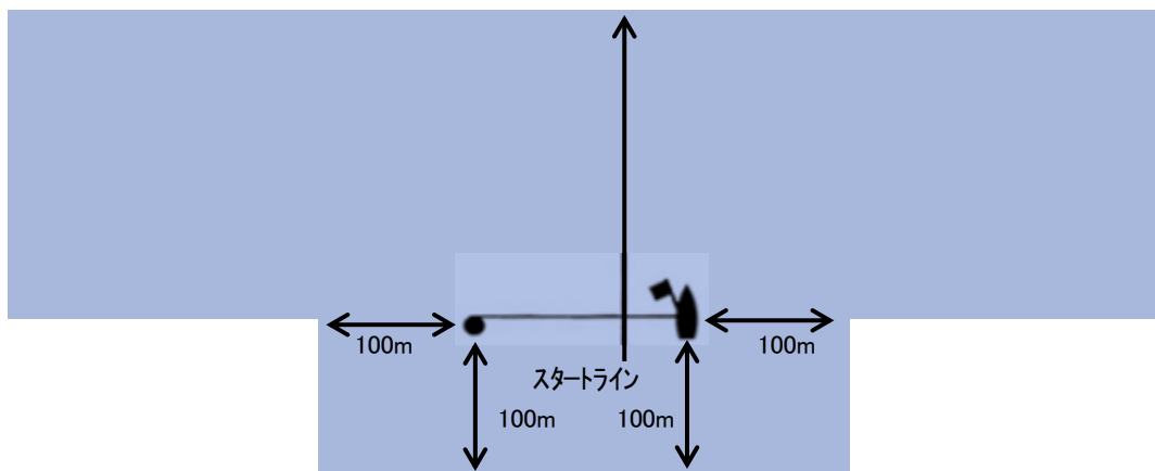
【添付図D】 指示10.4に規定するスタート・エリア
